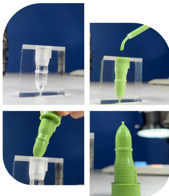
Exemple d'utilisation du F20 pour du contrôle de forme interne complète
